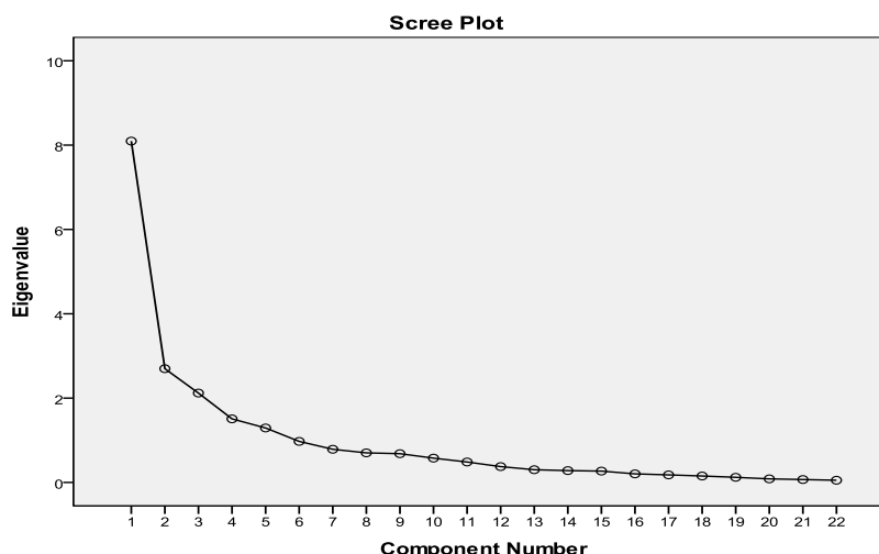
Gráfico 1 – Gráfico scree plot (análise fatorial 1)
