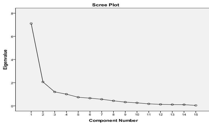
Gráfico 2 – Scree plot (análise fatorial 2)
