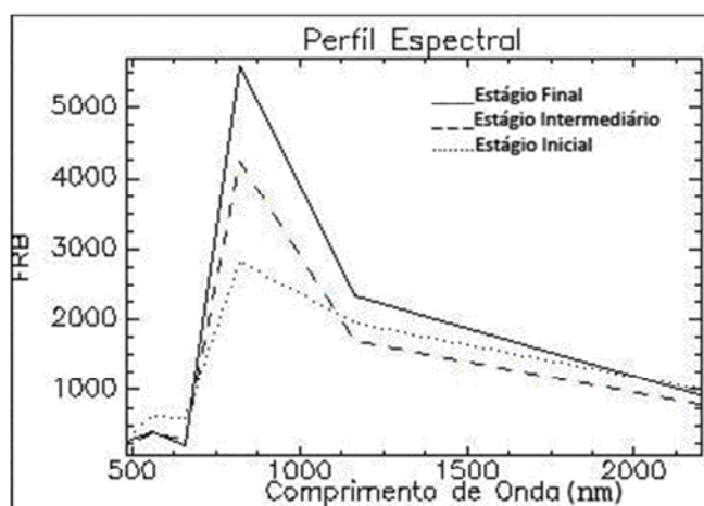
Figura 2. Dinâmica espectral exibida pela cultura da soja nas diferentes fases de desenvolvimento fenológico na imagem do sensor TM/Landsat-5.
